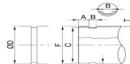
Fig. 5: 二端接頭凹槽尺寸時標示
