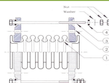
Fig. 6: 產品結構圖 口徑: 14" (含)以下
