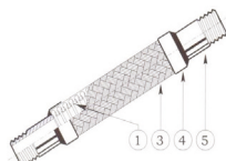
Fig. 2: JF-500T 結構圖
