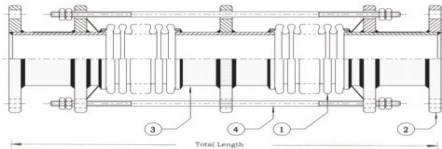
圖 2. 本結構為橫向位移: 大於 \pm 25 mm 構造。
