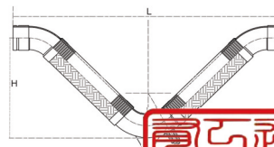
Fig. 11: 軟管左端固定，軟管右端能作：上下、左右移動使用。
