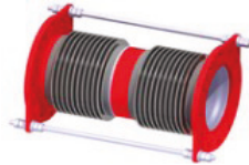
圖 1. 本結構為橫向位移: \pm 50 mm 構造。
