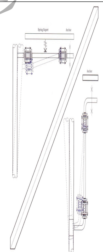
Fig. 26: 立管與水平分枝管之安裝設置。
