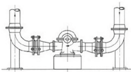
Fig. 29: 利用二防震接頭相互抵消作用力, 於此配管狀態下, 可調整防震接頭旁設限拉桿, 並將末端二顆螺帽反還緊。
