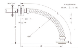
Fig. 10: 軟管左端固定、軟管右端端能作上下、左右移動使用。
