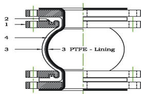
圖1. 產品結構圖
