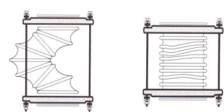
Fig. 37: 請選擇正確耐壓等級。上列圖式為耐壓不足狀態。
