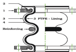
圖 1. 產品結構圖
