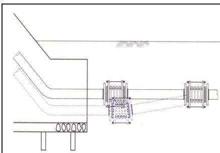
Fig. 18: 水管橋，吸收管路與建築物下沉位移。
