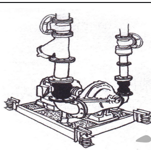
Fig. 5: 泵浦出、入口端，支撐架在防震基座上。
