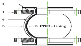
圖 1. 產品結構圖
