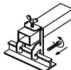
Fig. 7: T型鋼方管固定方式 -2
