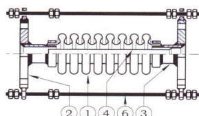
圖 1. JF-400SP、JF-400LSP 型產品外觀 圖 2. JF-400SPG、JF-400LSPG 型產品結構 圖 3. JF-400SG、JF-400LSG 型產品結構 圖 4. JF-400SG、JF-400LSG 型產品外觀
