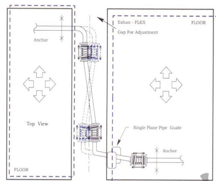
Fig. 22: 管路跨越伸縮縫，方式 (2)。
