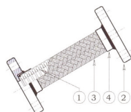
Fig. 2: 二端固定式法蘭產品結構圖
