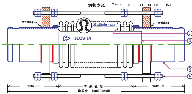
圖 1. JF-400 MSG、JF-400 LMSG 型產品結構
