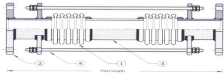
圖 1. 本結構為橫向位移: \pm 25 mm 構造。
