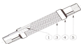
Fig. 2: ES-50T 結構 - 外牙式管牙
