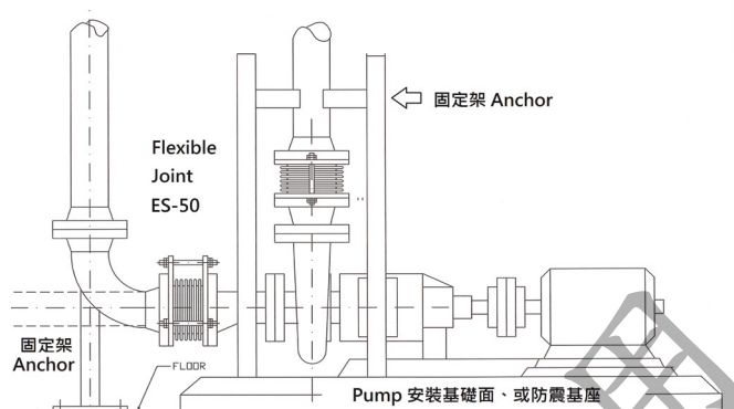
Fig. 28: 依上圖設置 Anchor 固定架(支撐點重量, 且不會產生位移。); 此配管狀態下, 可調整防震接頭旁設限拉桿, 並將末端二顆螺帽反還緊。
