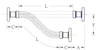
Fig. 8: 虛線為軟管安裝方式、實線為軟管動作。
