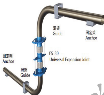
Fig. 3 : 應依配管需求，設置固定架( 固定管路不動 )、滑架 ( 可支撐管路重量，並固定管路移動、作動方向 )。
