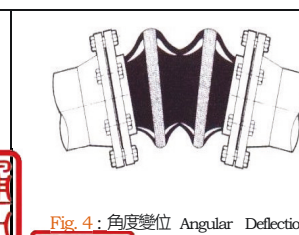
Fig. 4: 角度變位 Angular Deflection
