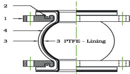
圖 1. 產品結構圖
