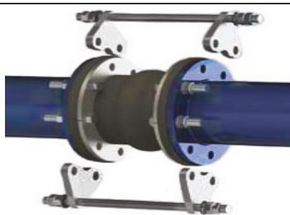
Fig. 1: 設限拉桿安裝前。
