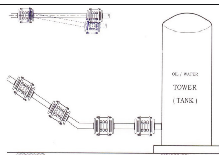
Fig. 20: 貯水槽、水塔：因負荷重、或地層鬆軟導致下陷。
