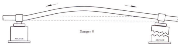
圖 1. 未安裝伸縮接頭（膨脹接頭），會因熱膨脹力無法消除，而使管路固定架負載增加，而產生彎曲變形、或掛齊管路固定架 Anchor、接頭焊合處、或周邊設備，會受此掛齊而產生洩漏、或毀損。
