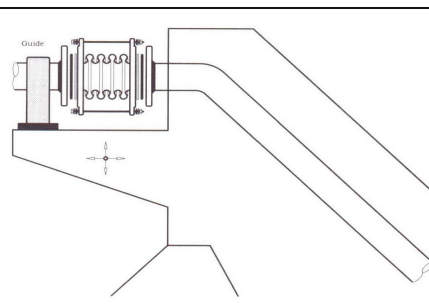
Fig. 19: 水管橋，可吸收因溫度變化伸縮及車輛行駛振動。
