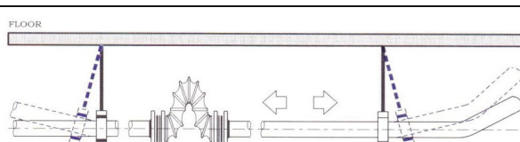
Fig. 36: 使用無設限拉桿型時, 應在適當位置安裝滑架與固定架。
