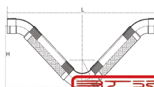
Fig. 5: 軟管左端固定，軟管右端僅能作：上下、左右移動使用。
