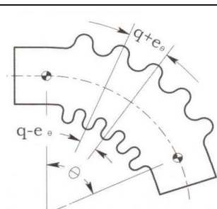
Fig. 39: 伸縮管二端受外力, 而產生“ \theta ”角度變位, 各山亦會產生相同變化, 因此, 當變化角度較大時, 其最高使用壓力必需降低。
