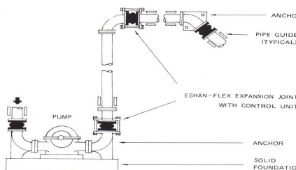
Fig. 9: 泵浦出、入口端，支撐架在防震基座上。
