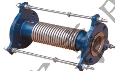
圖 4. JF-150 SG 型產品外觀（設限拉桿型）
