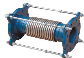
圖 1. JF-250SP、JF-250LSP 型產品外觀 圖 2. JF-250SPG、JF-250LSPG 型產品結構 圖 3. JF-250SG、JF-250LSG 型產品結構 圖 4. JF-250SG、JF-250LSG 型產品外觀
