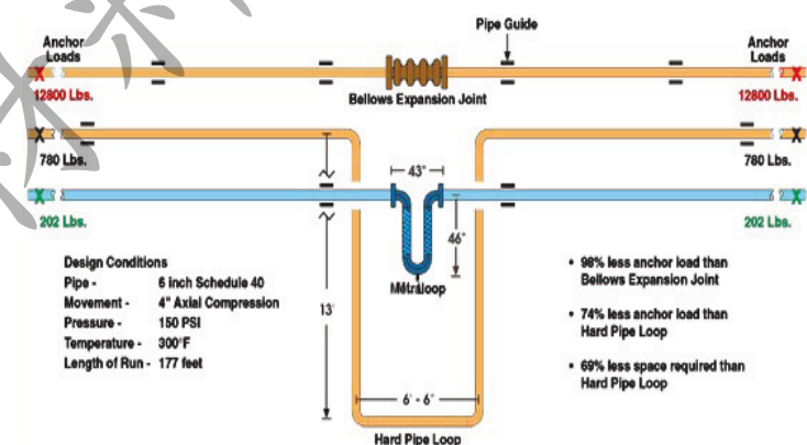
Fig. 6: U型軟管配管；可作一般件縮接頭使用，吸收管路熱脹冷縮，如上圖例。
