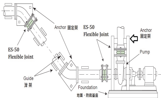
Fig. 27: Anchor 固定架(支撐點重量, 且不會產生位移。); Guide 滑架(支撐點重量, 並易於位移。); 此配管狀態下, 可調整防震接頭旁設限拉桿, 並將末端二顆螺帽反還緊。
