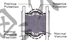
Fig. 1 : 軸向壓縮 AXIAL Compression
