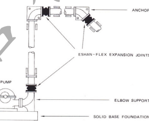
Fig. 11: 泵浦出、入口端，支撐架在防震基座上。
