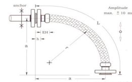
Fig. 10: 軟管左端固定、軟管右端端能作上下、左右移動使用。
