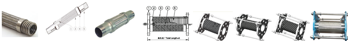
Fig. 1: 產品管體 Fig. 2: JF-500T 結構 Fig. 3: JF-500T 實體 Fig. 4: JF-600、JF-600H 產品結構及外觀 (設限拉桿依口徑, 決定支數)
