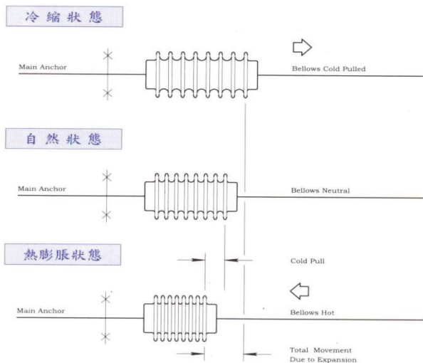
圖 2. 伸縮接頭與管路熱脹冷縮的互補關係
