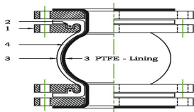
圖 1. 產品結構圖
