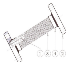
Fig. 2: JF-600 結構圖
