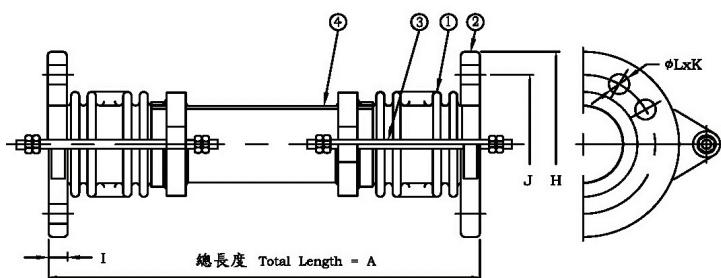
圖 1. 產品結構圖。
