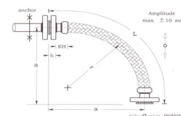
Fig. 4: 軟管左端固定，軟管右端僅能作：上下、左右移動使用。
