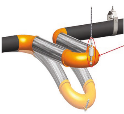
Fig. 8: U型配管方式；安裝參考。(可搭配任何接頭型式)
