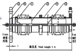
圖 2. 本結構為橫向位移: 大於 \pm 75 mm 構造。
