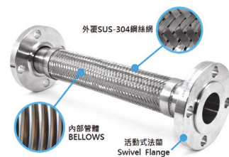
Fig. 3: 二端活動式法蘭產品結構圖
