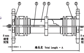
圖 2. 本結構為橫向位移：大於 +/- 75 mm 構造。
