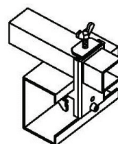
Fig. 3: C型鋼方管固定方式 -2
