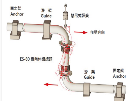
Fig. 2 : 應依配管需求，設置固定架、滑架、懸吊式彈簧。
