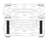
Fig. 5: 法蘭與伸縮管連接型 口徑: 14" (含)以上
