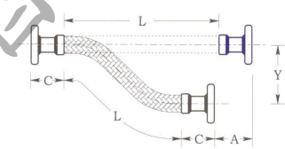
Fig. 2: 虛線為軟管安裝方式，實線為軟管作動。
