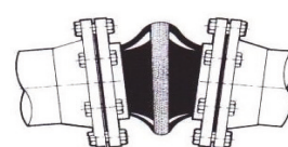
Fig. 4: 角度變位 Angular Deflection
