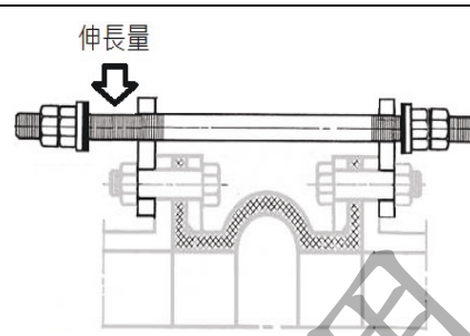
Fig. 3: 設限拉桿安裝後，螺帽距離調整【伸長量】，請參閱各型號之伸長量調整。
