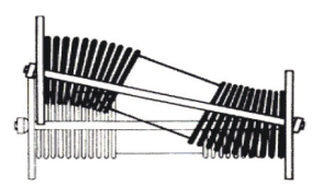
圖 3. 本產品橫向位移作動圖。
