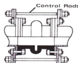
Fig. 2 : 軸向拉伸 Axial Extension
