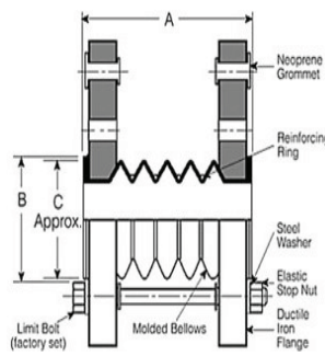
Fig. 5: 產品結構圖
