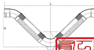
Fig. 11: 軟管左端固定、軟管右端端能作上下、左右移動使用。
