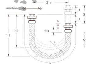
Fig. 1: 軟管不可作拉伸、或壓縮使用。
