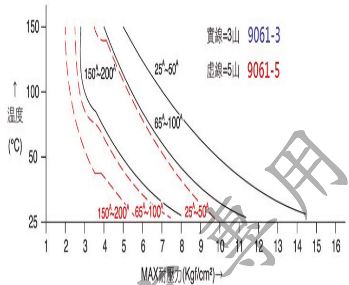
Fig. 6: 溫度與壓力曲線
