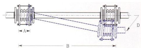
圖 2. 產品橫向位移作動圖。
