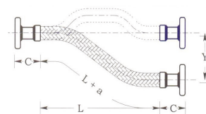
Fig. 9: 虛線為軟管安裝方式、實線為軟管動作。
