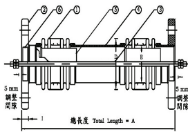
圖 1. 本結構為橫向位移: \pm 50 mm 構造。
