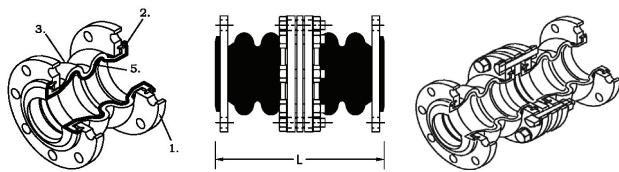
圖 1. ES-200 型爆炸圖結構
