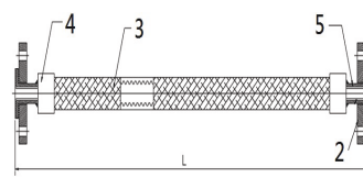
Fig. 3: 二端活動式法蘭產品結構圖
