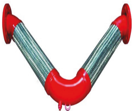
Fig. 3: V型最佳配管方式；V型不銹鋼軟管具有 X、Y、Z 三軸向位移作動。
