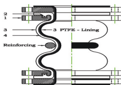
圖 1. 產品結構圖
