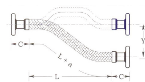
Fig. 3: 虛線為軟管安裝方式，實線為軟管作動。
