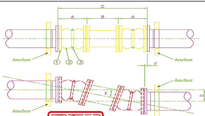
Fig. 13: 雙球型大位移量之安裝方式。
