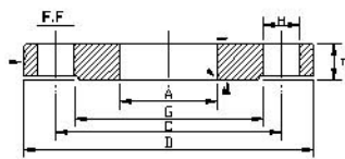
ANSI 125型 FLANGES
