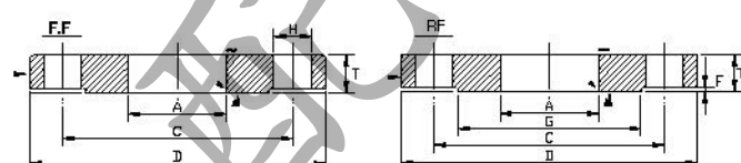
ANSI 300型 FLANGES
