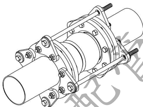
Installation Chart 管路安裝圖
