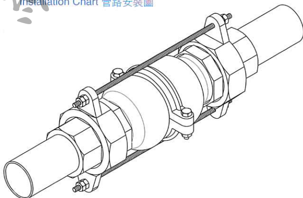
Installation Chart 管路安裝圖
