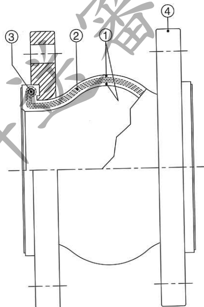
construction 產品結構圖
